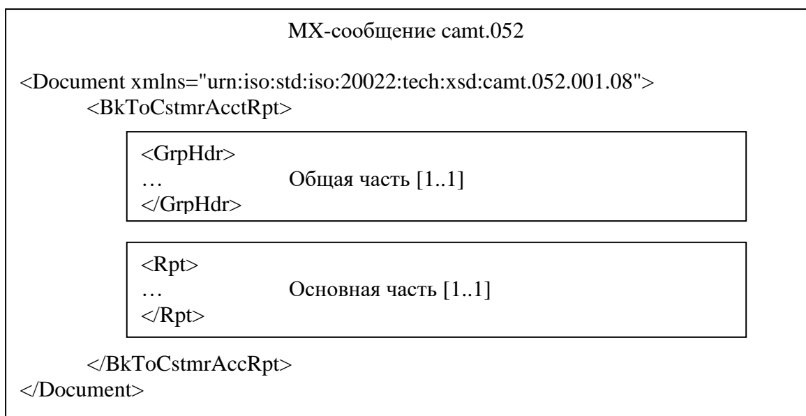
Рисунок 1 – Структура МХ-сообщения camt.052
